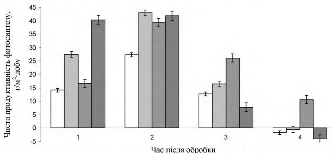
Рис. Вплив стимуляторів росту на чисту продуктивність фотосинтезу рослин картоплі сорту Санте (середні дані за 2013 і 2014 роки): час після обробки 1 – 1–10-та, 2 – 10–20-та, 3 – 20–30-та, 4 – 30–40-ва доба;
